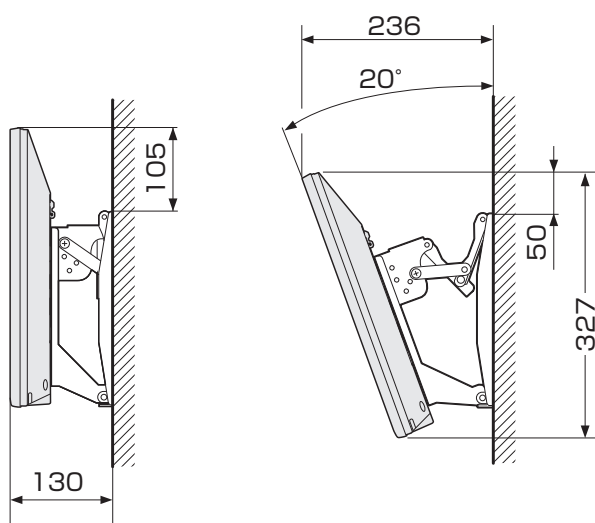
壁掛け金具AN-130AG1使用時
